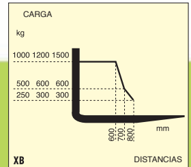
Diagrama de carga máxima en base a la altura
